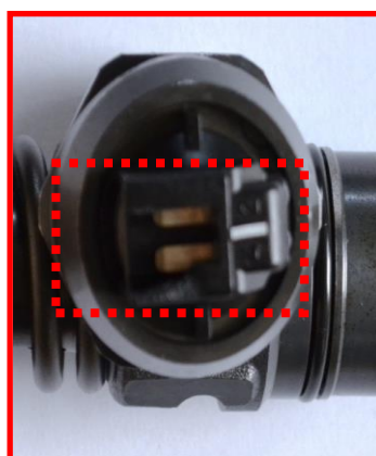
Poškozený konektor
